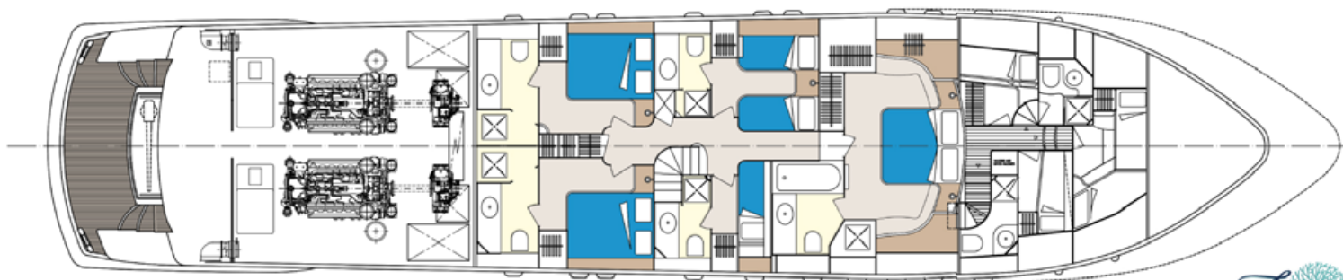
MAIORA 31: LOWER DECK PLAN (SC. 1/50)
